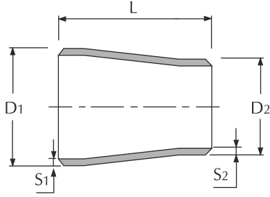
KONSANTRİK / CONS
