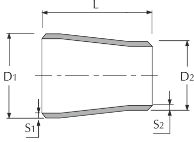
KONSANTRİK
