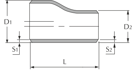
EKSANTRİK / ECC
