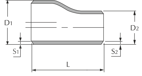
EKSANTRİK
